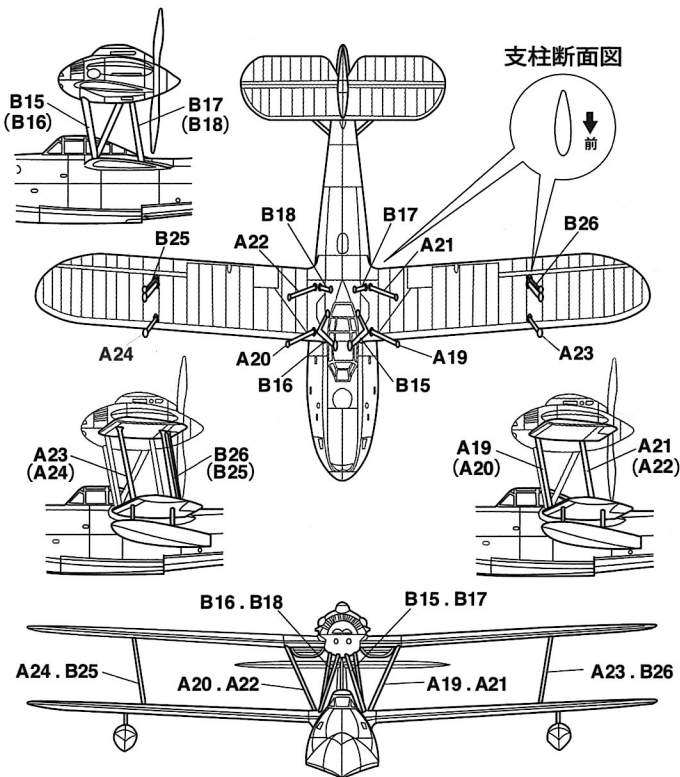
支柱取付図
