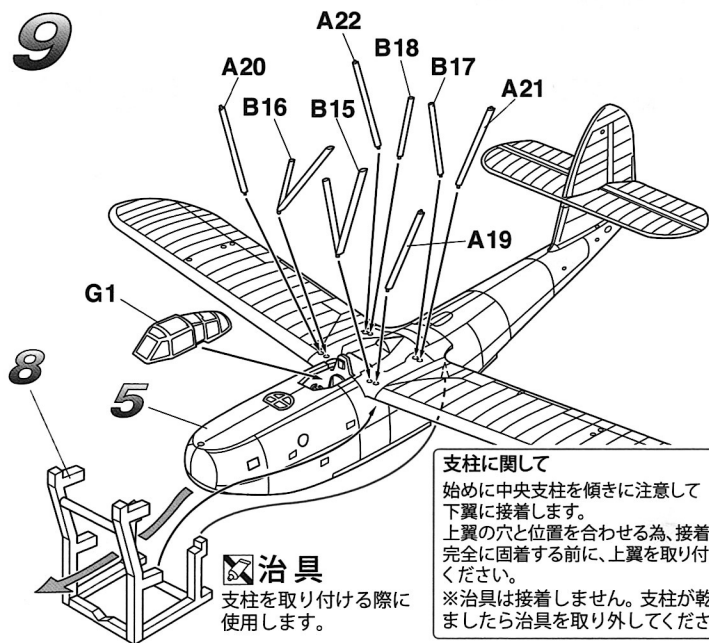
支柱取付図
